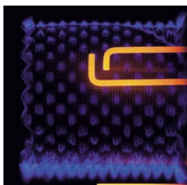
Quemador cilíndrico Matrix de muy bajas emisiones
