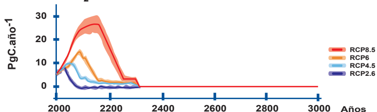
Concentración CO 2 atmósfera
