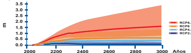
Expansión térmica del océano
