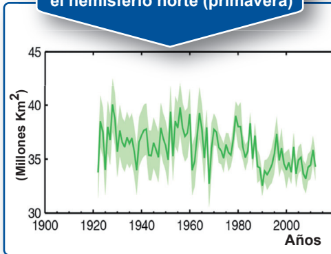
Cobertura de nieve en el hemisferio norte (primavera)
