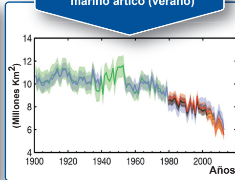
Extensión del hielo marino ártico (verano)
