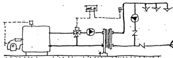
FIG.12.-INSTALACION EXCLUSIVA DE ACS CON INTERCAMBIADOR
